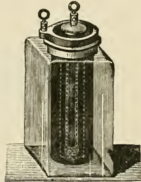
FIG. 101. — Léclanche cell.
